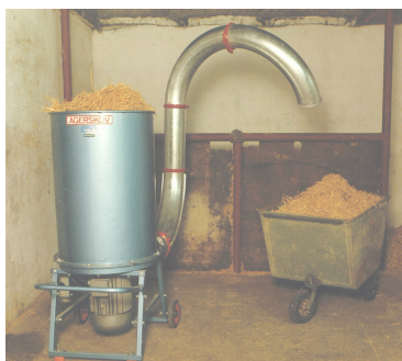
AM 35 SU Fixe à introduction verticale. Règlable dans la direction de projection d'épandage désirés. Moteur électrique 10 cv.
